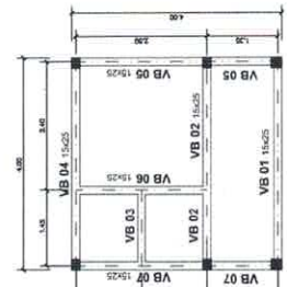
PLANTA DE FORMAS FUNDAÇÃO - VIGAS BALDRAME ESC. 1/50
