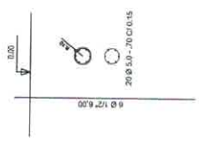
ESTACA - E1, E2, E3, E4, E5, E6, E7, E8, E9, E11, E12, E13, E14, E15, E16, E17, E18 PLANTA E CORTE - ESC. 1/25
