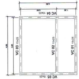
PLANTA DE FORMAS COBERTURA ESC. 1/50
